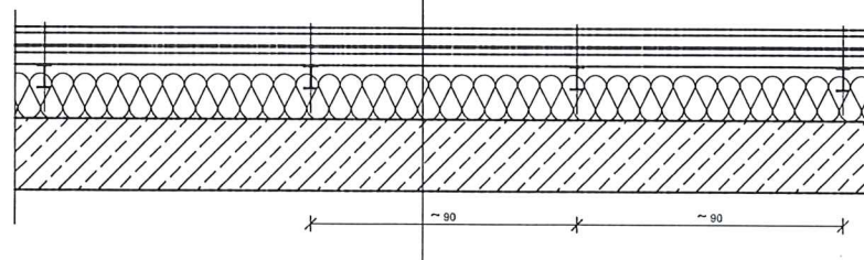
PRZEKRÓJ A-A
