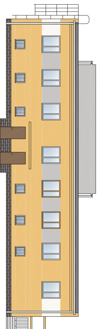
ELEWACJA ZACHODNIA
