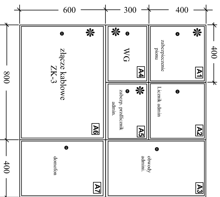
Proj. rozdzielnia główna TG1/TA - kl.schod. K-1
