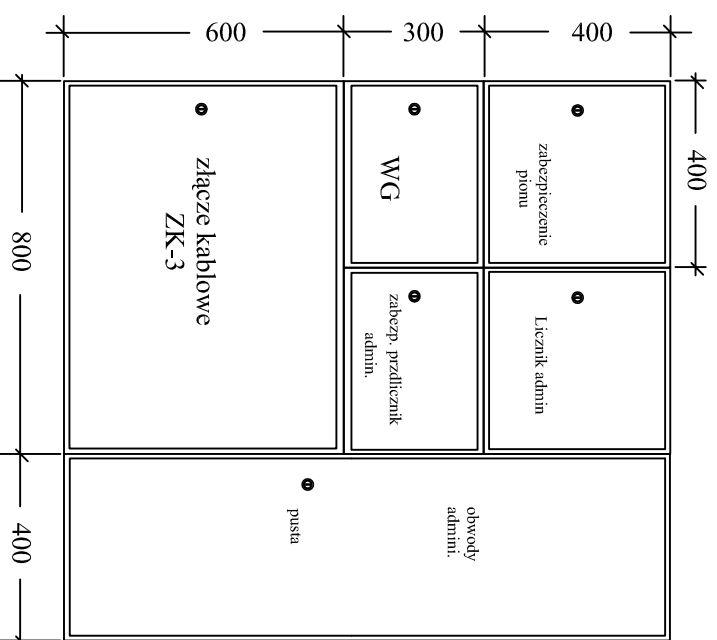
Istn. rozdzielnia główna TG1/TA - kl.schod. K-1
