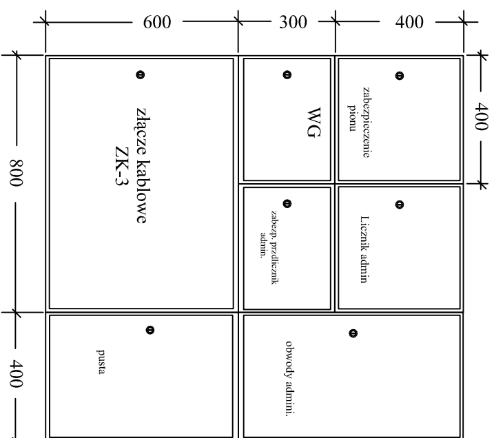
Istn. rozdzielnia główna TG2/TA - Kl.schod. K-2
