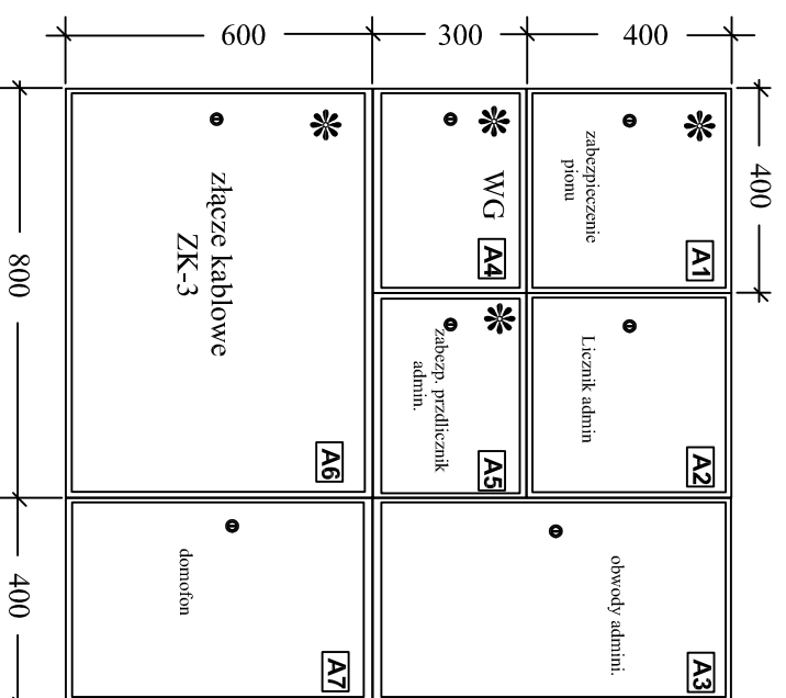
Proj. rozdzielnia główna TG2/TA - Kl.schod. K-2
