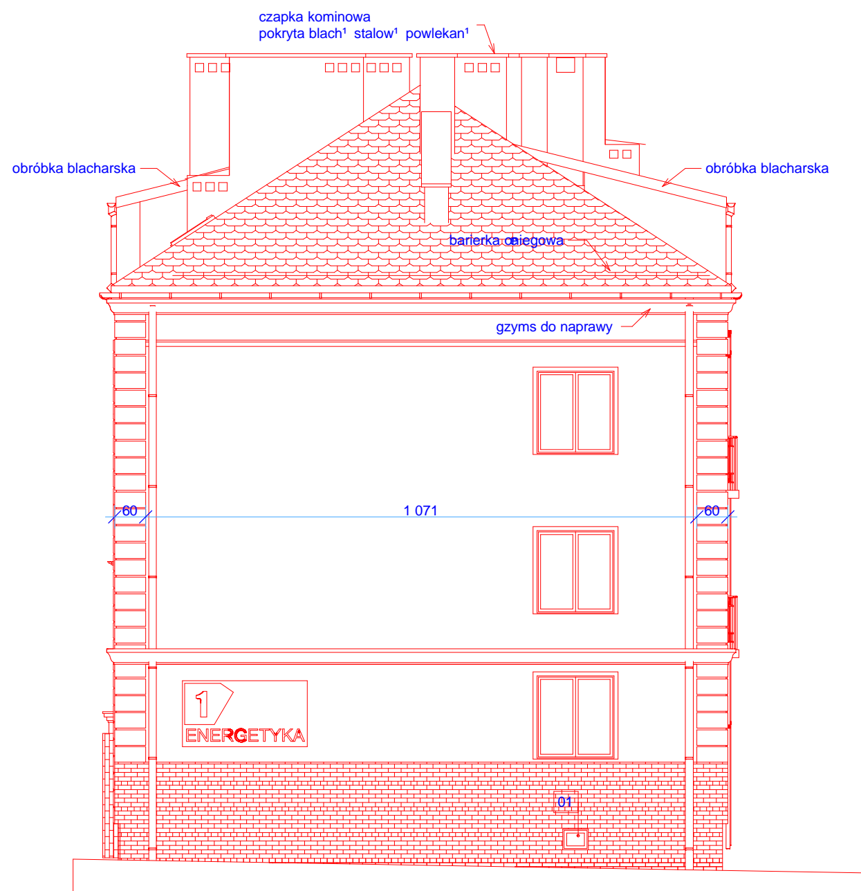
Elewacja południowa
