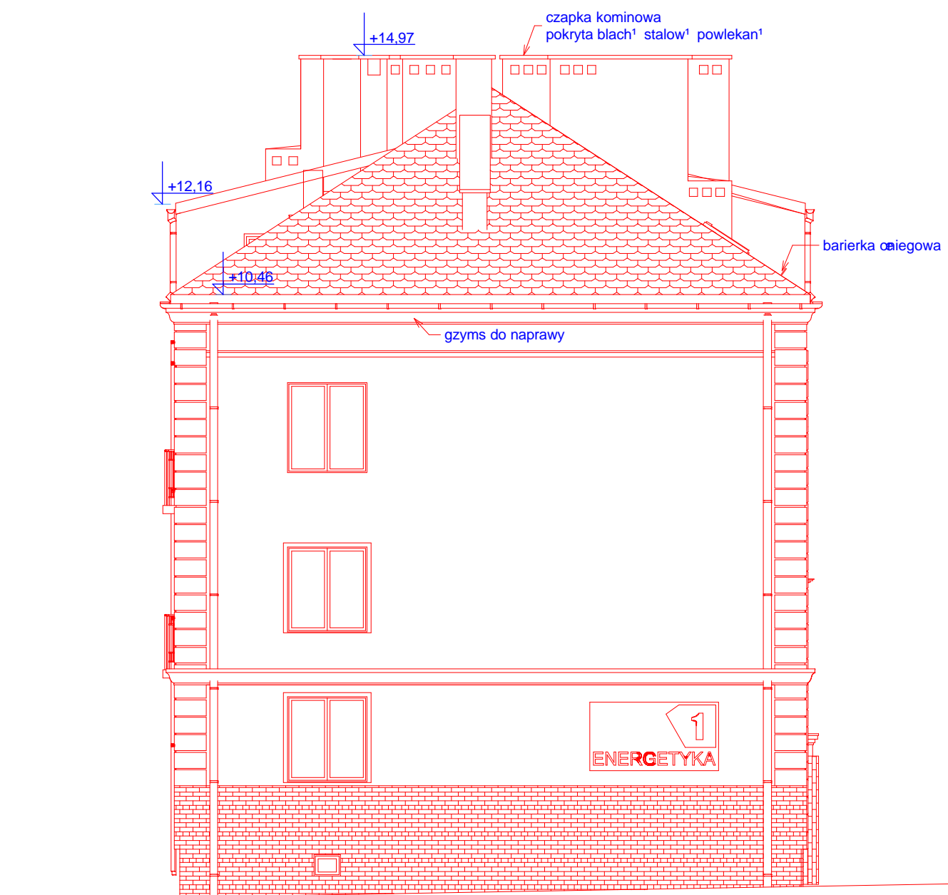
Elewacja północna
